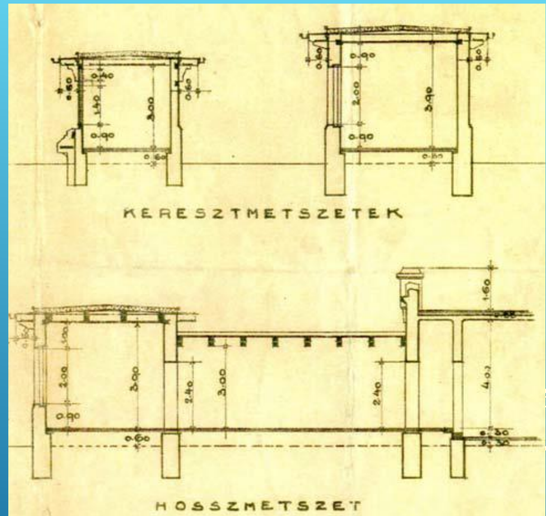
AZ EREDETI TERV METSZETEI
