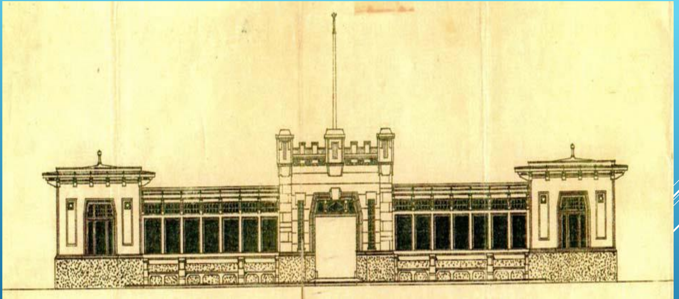
A VÍZPARTI HOMLOKZAT – KAÁLI NAGY EREDETI TERVE
